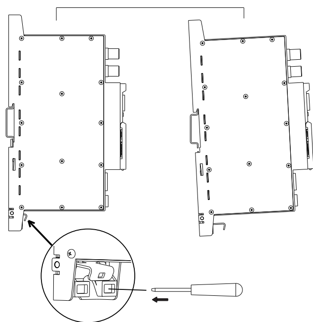
Рис. 4. Демонтаж с планки "DIN rail"
