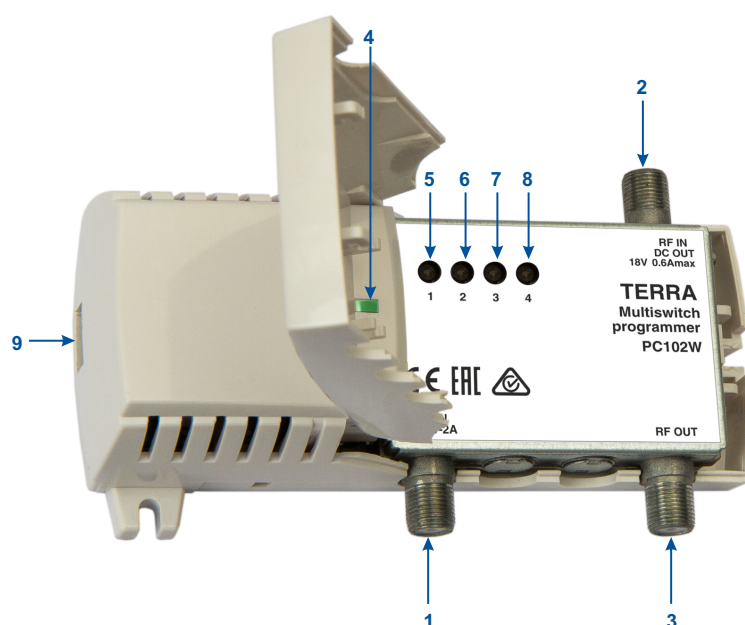
Rysunek 1. Wygląd zewnętrzny programatora z oznaczeniem jego elementów
