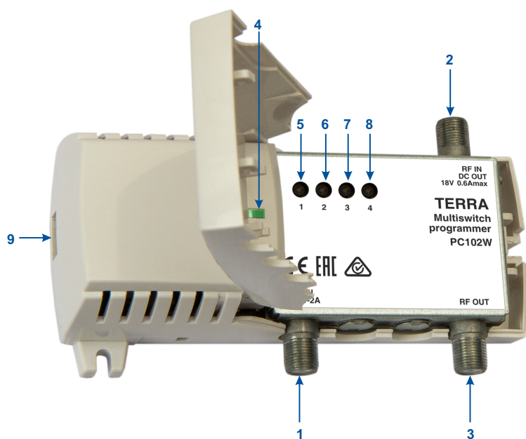
Рис. 1. Внешний вид программатора
