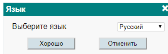
Рис. 28. Выбор языка
